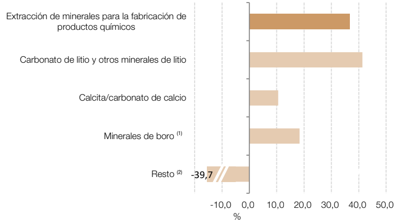
Gráfico 4.5.2 Extracción de minerales para la fabricación de productos químicos, variación porcentual interanual. Abril de 2025
