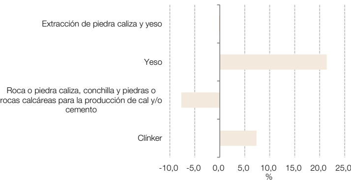
Gráfico 4.2.2 Extracción de piedra caliza y yeso, variación porcentual interanual. Abril de 2025
