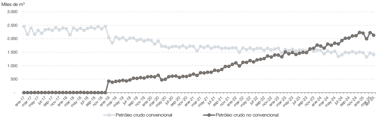
Gráfico 6.2 Extracción de petróleo crudo convencional y no convencional, en miles de m³. Enero 2017-abril 2025
