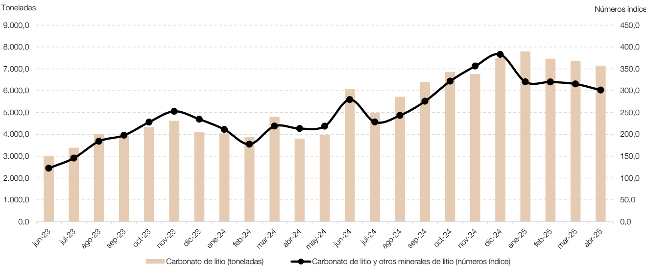
Gráfico 8. Carbonato de litio y otros minerales de litio, en toneladas y números índice. Junio 2023-abril 2025
