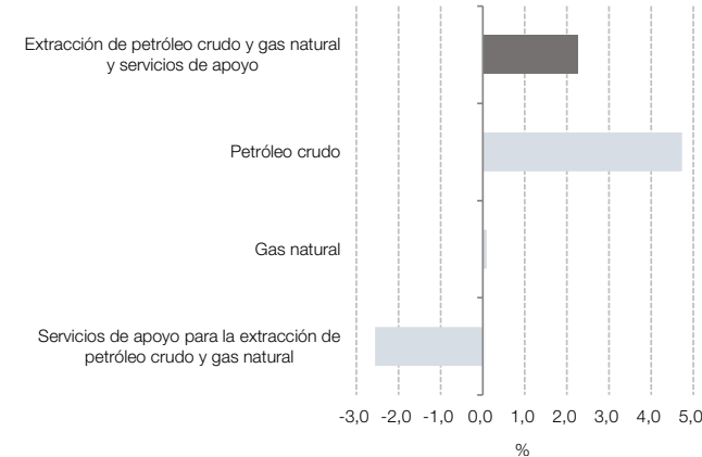
Gráfico 2.3 Petróleo crudo, gas natural y servicios de apoyo, incidencias. Abril de 2025
