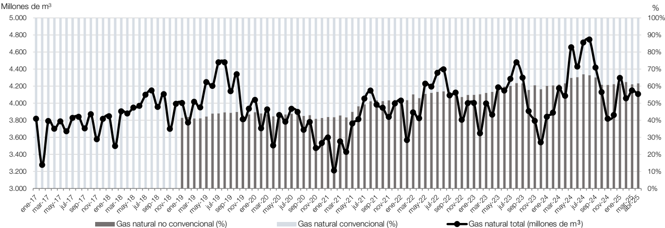
Gráfico 7.1 Extracción de gas natural convencional y no convencional, en millones de m³ y estructura porcentual. Enero 2017-abril 2025
