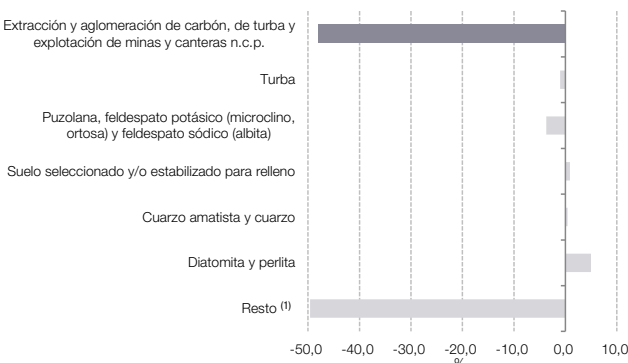
Gráfico 4.7.3 Carbón, turba y explotación de minas y canteras n.c.p., incidencias. Abril de 2025
