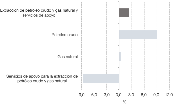
Gráfico 2.2 Petróleo crudo, gas natural y servicios de apoyo, variación porcentual interanual. Abril de 2025
