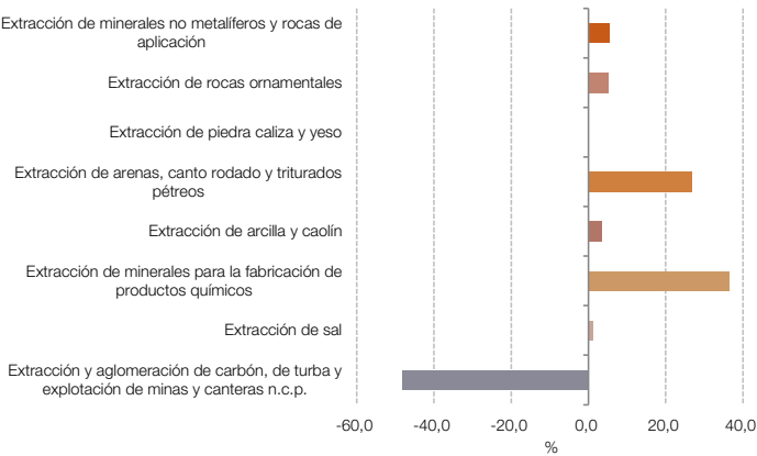
Gráfico 4.2 Minerales no metalíferos y rocas de aplicación, variación porcentual interanual. Abril de 2025
