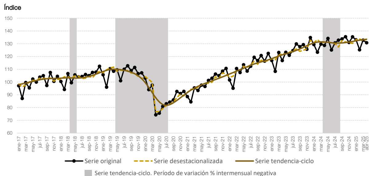
Gráfico 1.1 IPI minero nivel general. Serie original, desestacionalizada y tendencia-ciclo, base 2016=100, en números índice. Enero 2017-abril 2025
