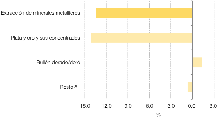
Gráfico 3.3 Extracción de minerales metalíferos, incidencias. Abril de 2025
