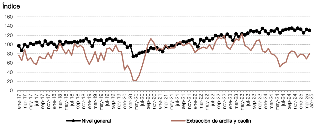
Gráfico 4.4.1 Extracción de arcilla y caolín respecto al nivel general del IPI minero, en números índice. Enero 2017-abril 2025
