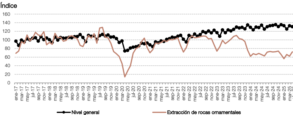
Gráfico 4.1.1 Extracción de rocas ornamentales respecto al nivel general del IPI minero, en números índice. Enero 2017-abril 2025
