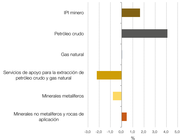
Gráfico 1.3 IPI minero nivel general y categorías, incidencias. Abril de 2025
