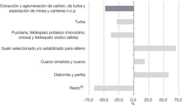
Gráfico 4.7.2 Carbón, turba y explotación de minas y canteras n.c.p., variación porcentual interanual. Abril de 2025
