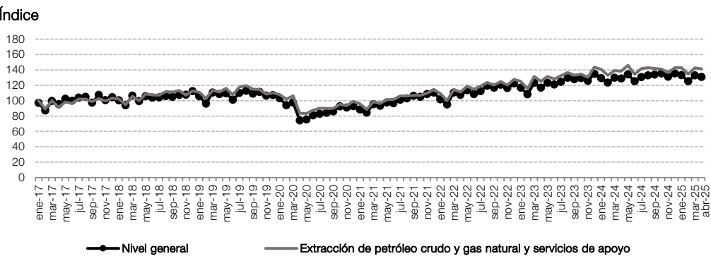
Gráfico 2.1 Extracción de petróleo crudo y gas natural y servicios de apoyo respecto al nivel general del IPI minero, en números índice. Enero 2017-abril 2025
