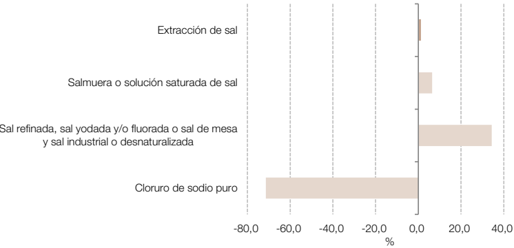
Gráfico 4.6.2 Extracción de sal, variación porcentual interanual. Abril 2025
