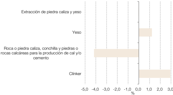
Gráfico 4.2.3 Extracción de piedra caliza y yeso, incidencias. Abril de 2025
