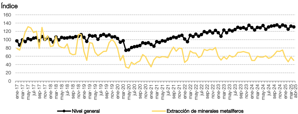
Gráfico 3.1 Extracción de minerales metalíferos respecto al nivel general del IPI minero, en números índice. Enero 2017-abril 2025
