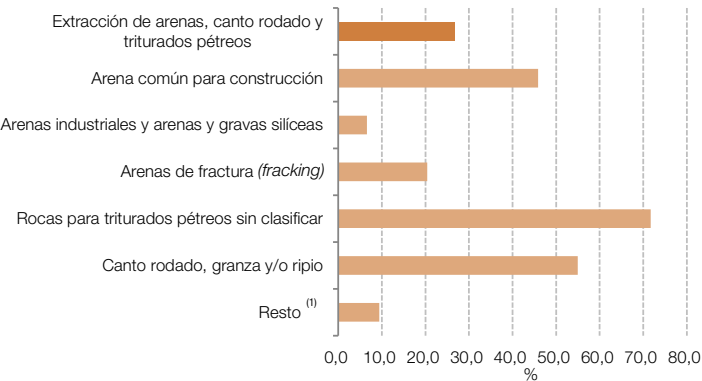
Gráfico 4.3.2 Extracción de arenas, canto rodado y triturados pétreos, variación porcentual interanual. Abril de 2025
