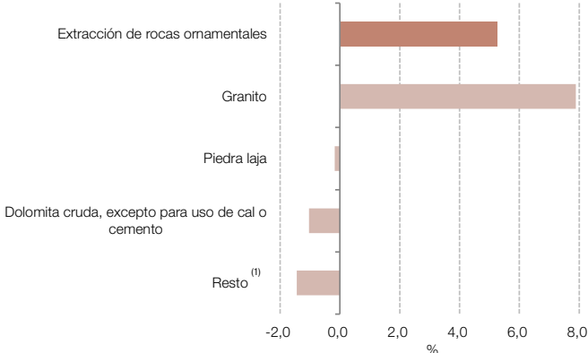
Gráfico 4.1.3 Extracción de rocas ornamentales, incidencias. Abril de 2025
