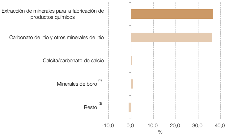
Gráfico 4.5.3 Extracción de minerales para la fabricación de productos químicos, incidencias. Abril de 2025
