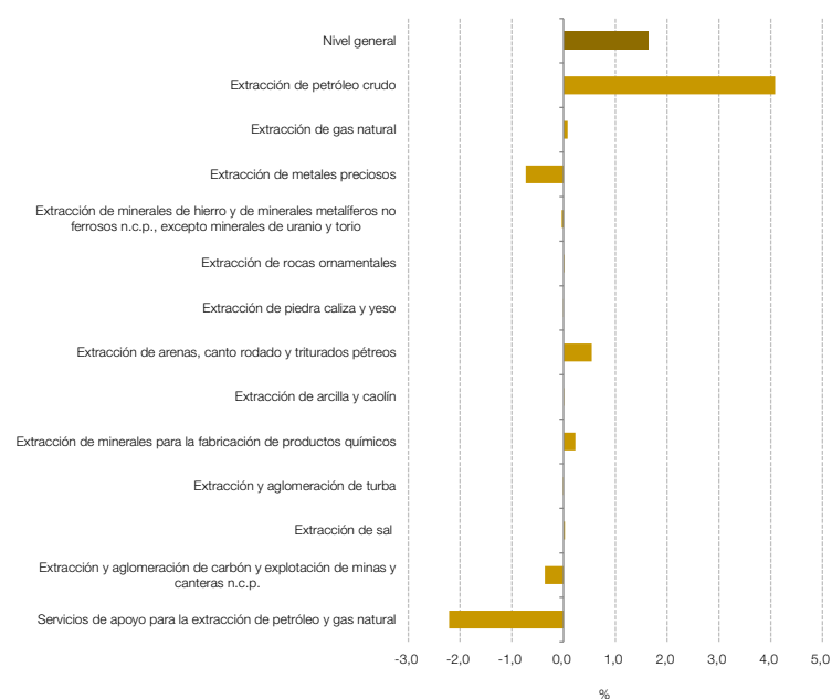
Gráfico 5.2 IPI minero nivel general y subclases, incidencias. Abril de 2025
