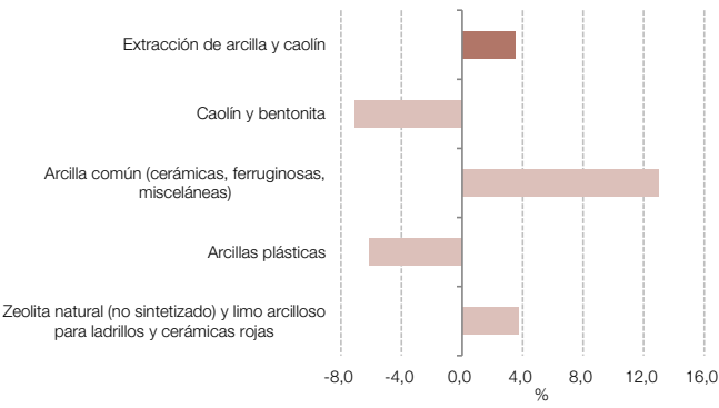
Gráfico 4.4.3 Extracción de arcilla y caolín, incidencias. Abril de 2025
