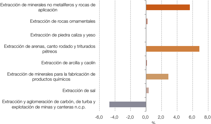
Gráfico 4.3 Minerales no metalíferos y rocas de aplicación, incidencias. Abril de 2025
