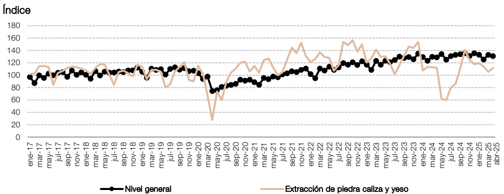
Gráfico 4.2.1 Extracción de piedra caliza y yeso respecto al nivel general del IPI minero, en números índice. Enero 2017-abril 2025
