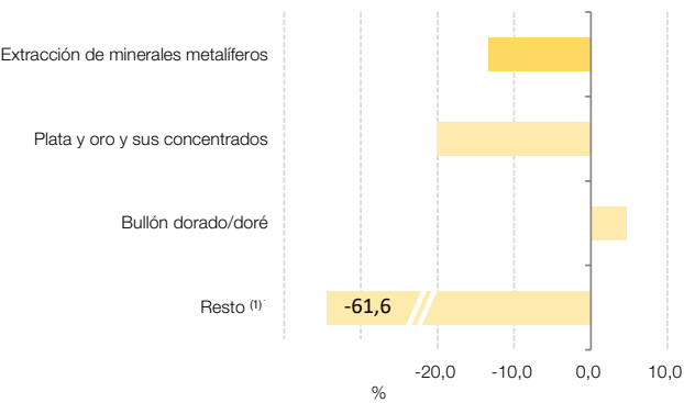
Gráfico 3.2 Extracción de minerales metalíferos, variación porcentual interanual. Abril de 2025
