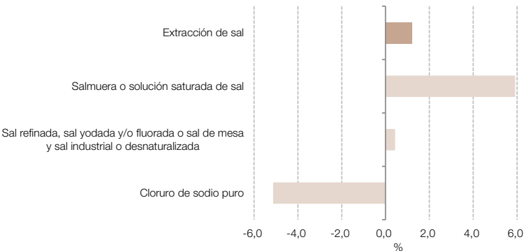
Gráfico 4.6.3 Extracción de sal, incidencias. Abril 2025
