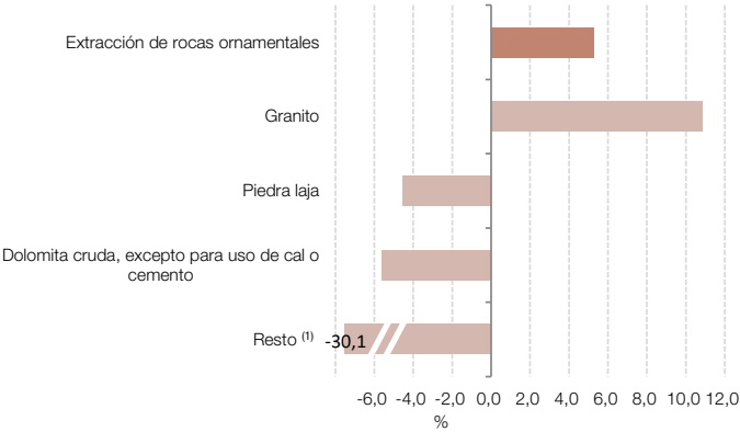
Gráfico 4.1.2 Extracción de rocas ornamentales, variación porcentual interanual. Abril de 2025
