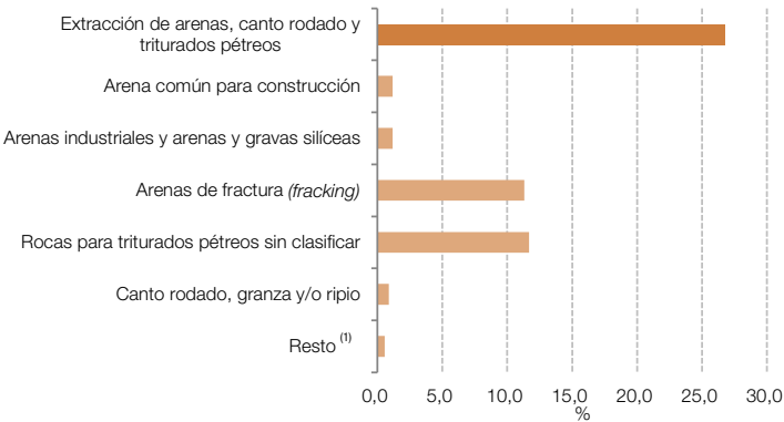
Gráfico 4.3.3 Extracción de arenas, canto rodado y triturados pétreos, incidencias. Abril de 2025
