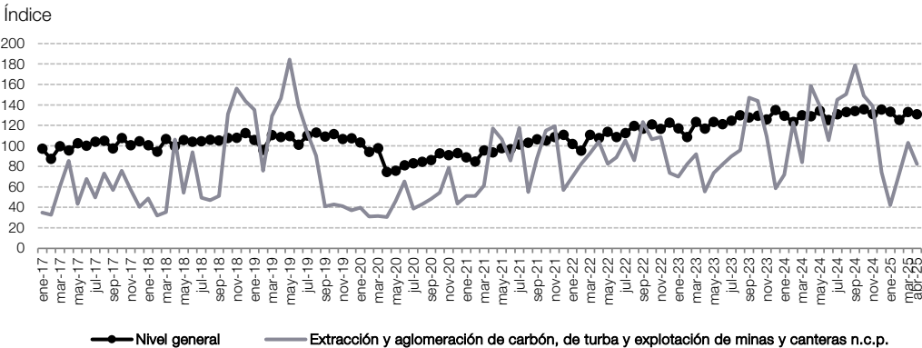
Gráfico 4.7.1 Extracción y aglomeración de carbón, de turba y explotación de minas y canteras n.c.p. respecto al nivel general del IPI minero, en números índice. Enero 2017-abril 2025
