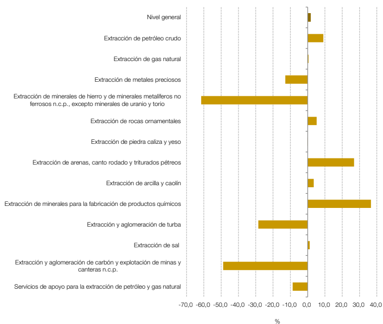
Gráfico 5.1 IPI minero nivel general y subclases, variación porcentual interanual. Abril de 2025
