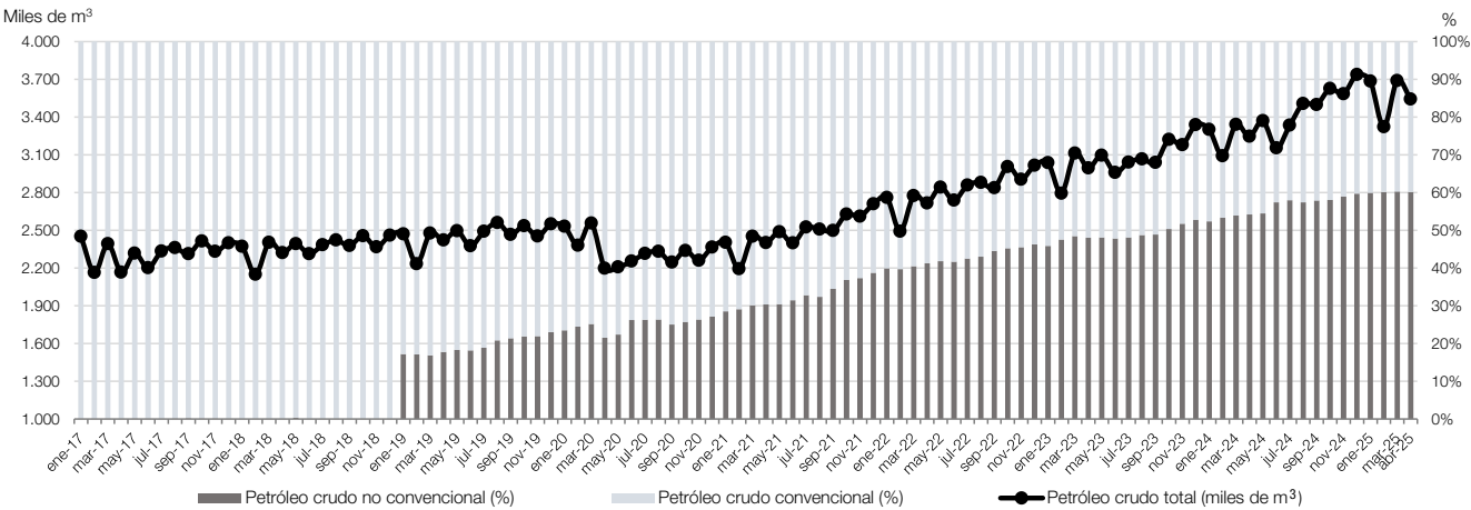
Gráfico 6.1 Extracción de petróleo crudo convencional y no convencional, en miles de m³ y estructura porcentual. Enero 2017-abril 2025
