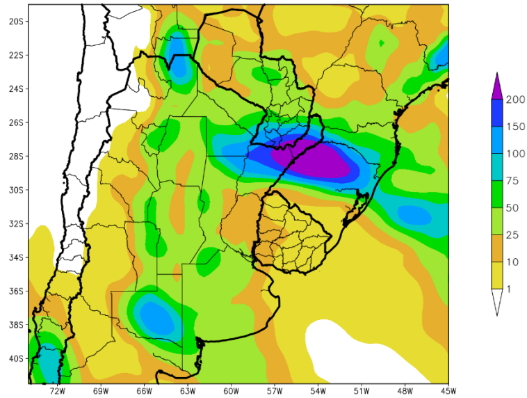
PERSPECTIVA DEL 10 AL 16 DE NOVIEMBRE DE 2022 PRECIPITACION (mm)
