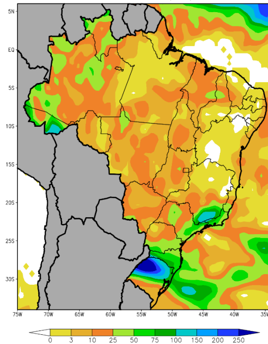
PERSPECTIVA DEL 10 AL 16 DE NOVIEMBRE DE 2022 PRECIPITACION (mm)
