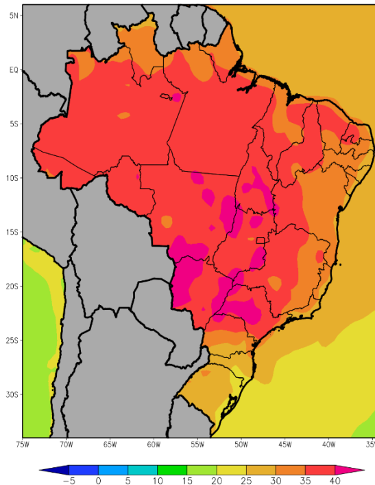
PERSPECTIVA DEL 10 AL 16 DE NOVIEMBRE DE 2022 TEMPERATURA MAXIMA(Grados Cent.)
