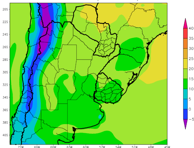
PERSPECTIVA DEL 10 AL 16 DE NOVIEMBRE DE 2022 TEMPERATURA MINIMA(Grados Cent.)
