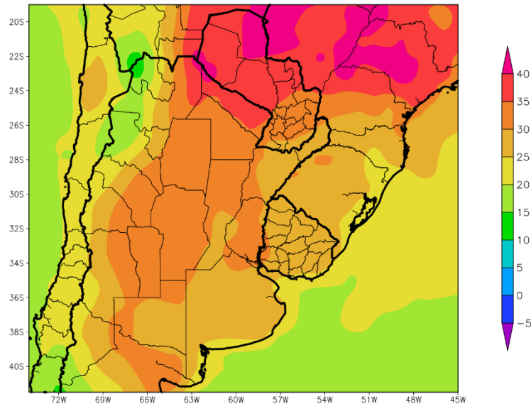
PERSPECTIVA DEL 10 AL 16 DE NOVIEMBRE DE 2022 TEMPERATURA MAXIMA(Grados Cent.)
